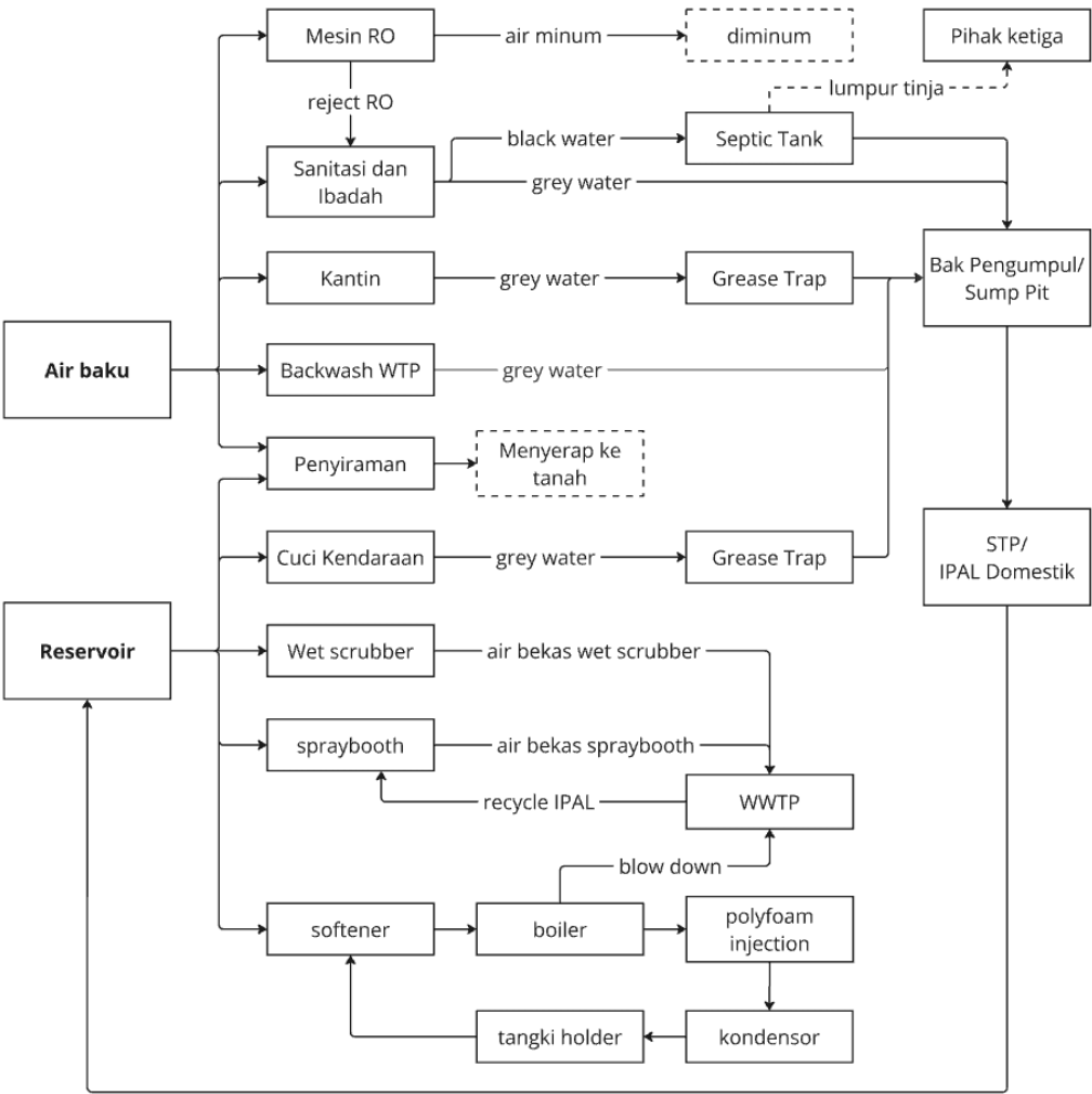
Gambar 4. Diagram Alir Pengelolaan Air Limbah Keseluruhan
