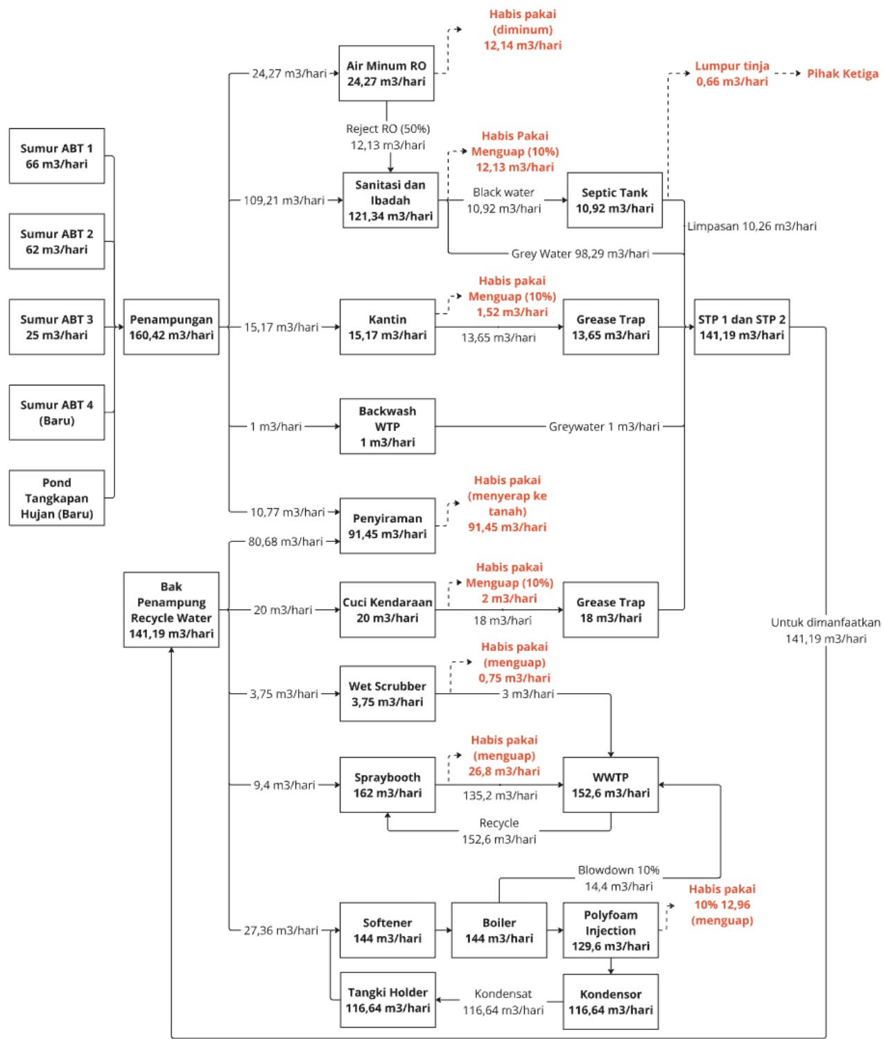
Gambar 1. Neraca Air Tahap Operasional
