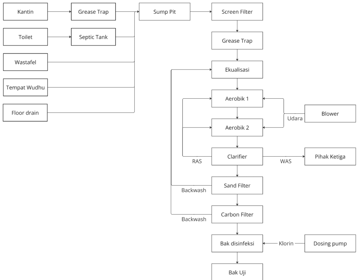
Gambar 6. Diagram Alir STP 2
