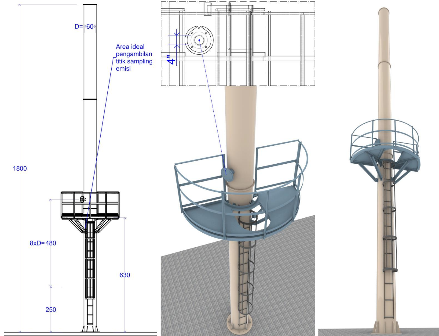
Gambar 4. Cerobong Boiler 1 dan 2
